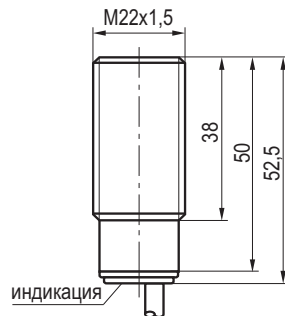
Габаритный чертеж
